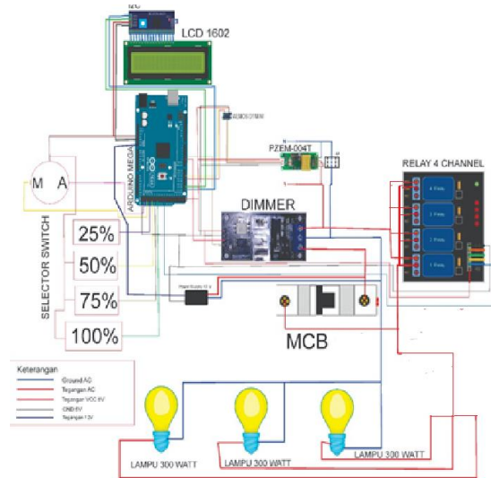
Gambar 5. Diagram Perancangan
