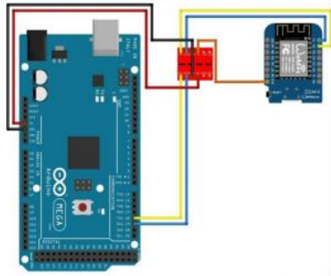
Gambar 7. Rangkaian Wemos D1 Mini Pro
